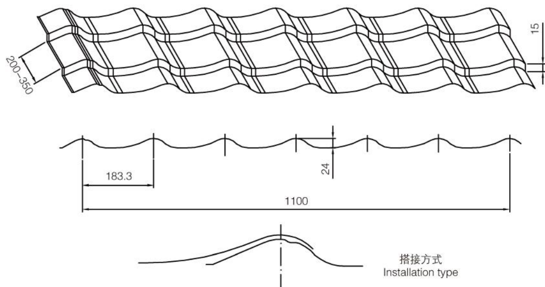
立体效果图 Stereo view
