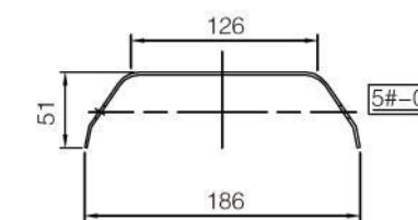
A—A 2:1
