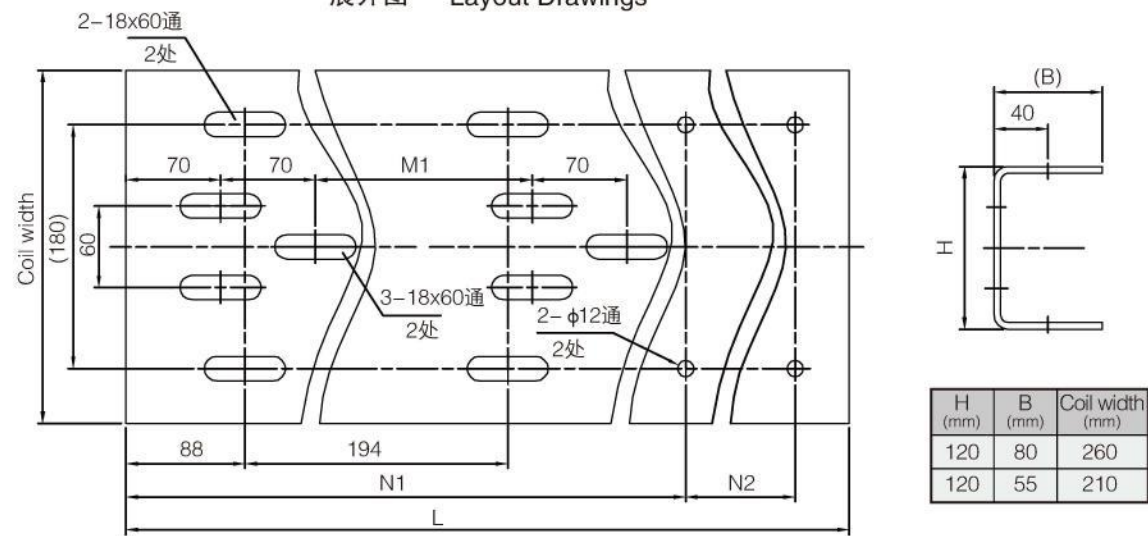
展开图 Layout Drawings
