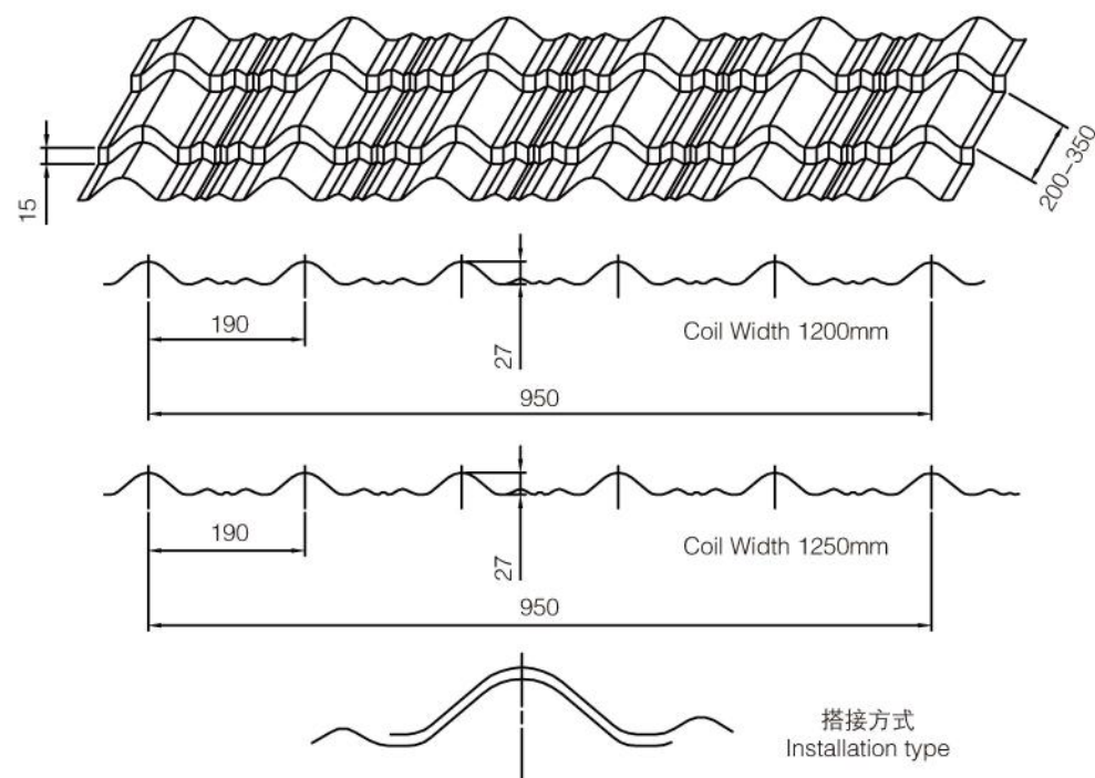
立体效果图 Stereo view
