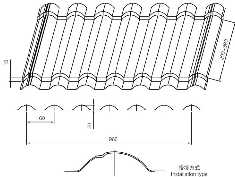
立体效果图 Stereo view
