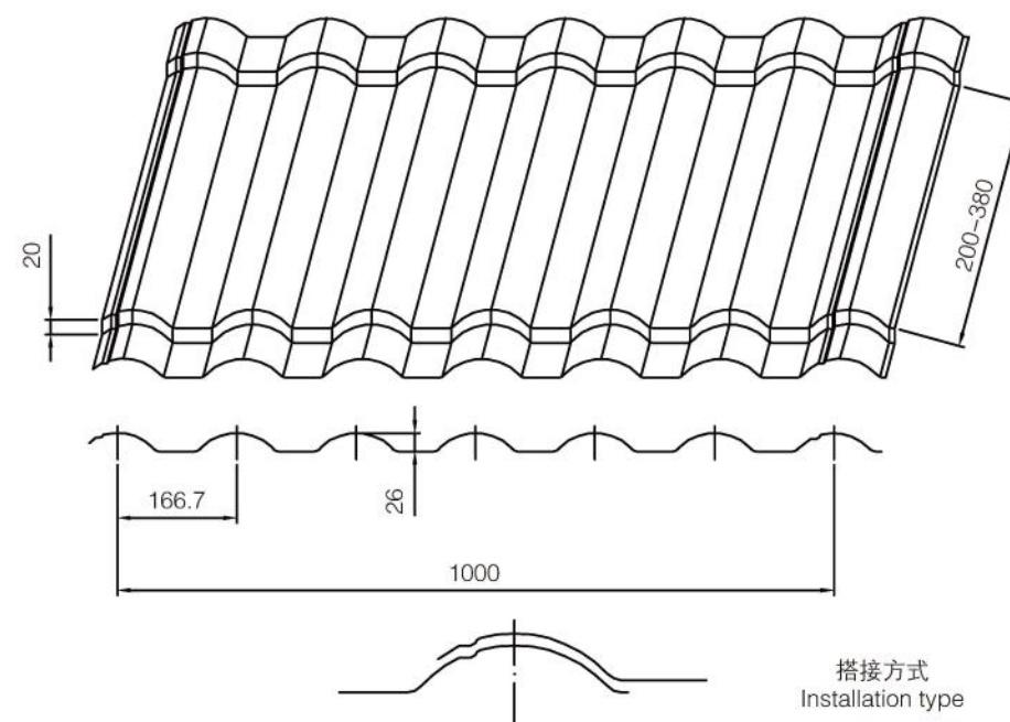
立体效果图 Stereo view
