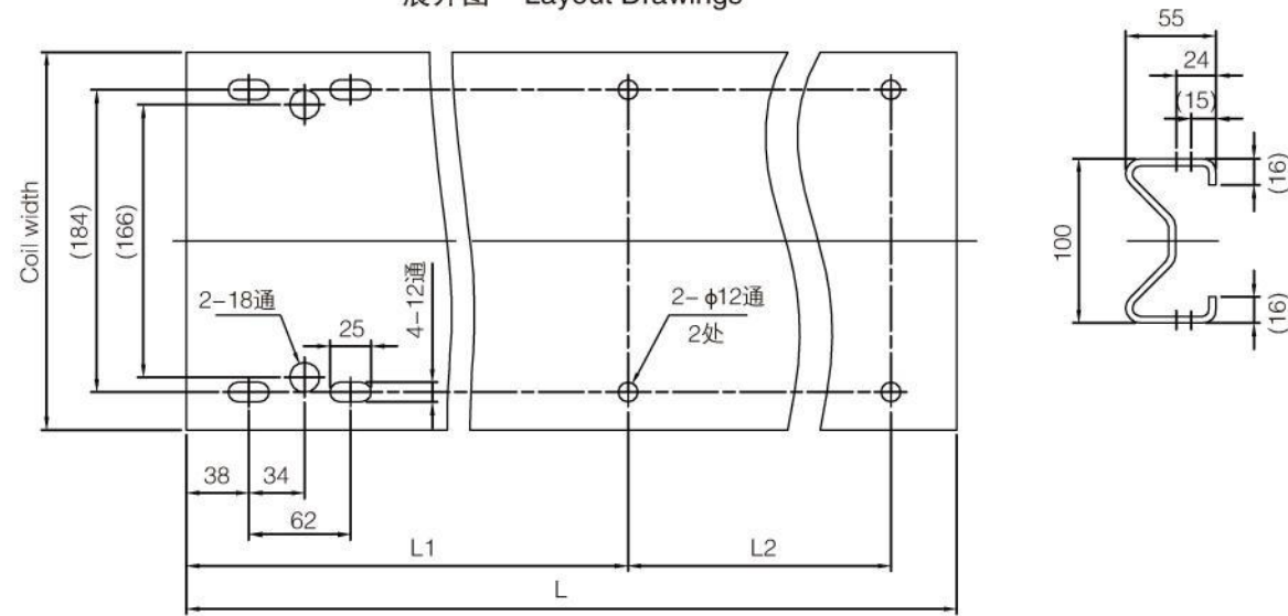
展开图 Layout Drawings
