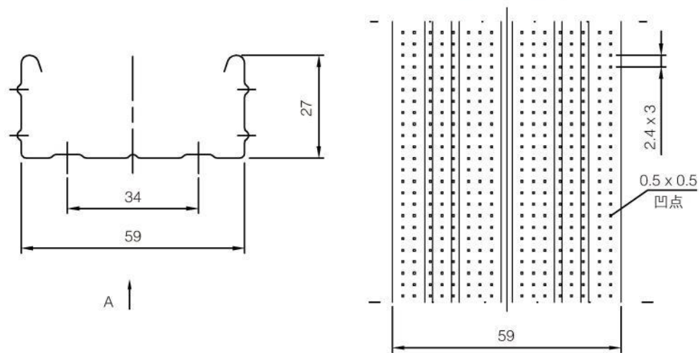
A向 底面压花图 Embossing drawings
